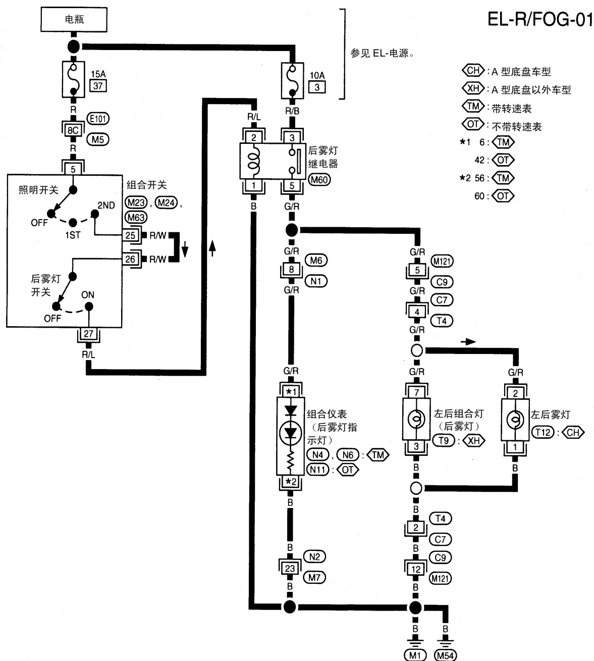
电路图 一 后雾灯 一/左舵车型
